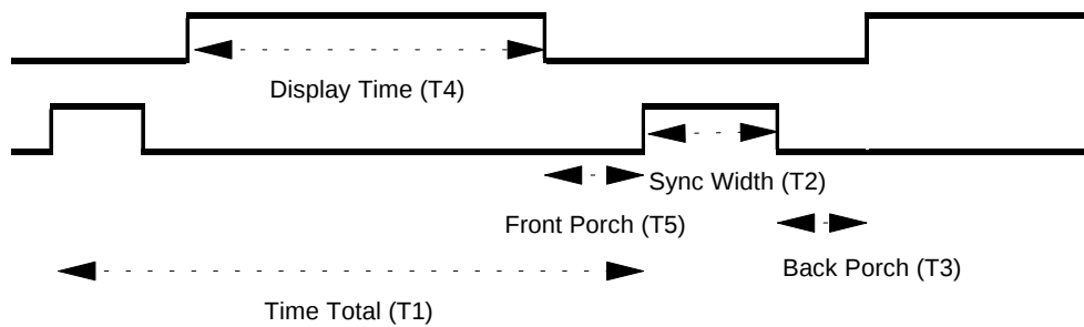
Fig. 3.03 - V-Sync
