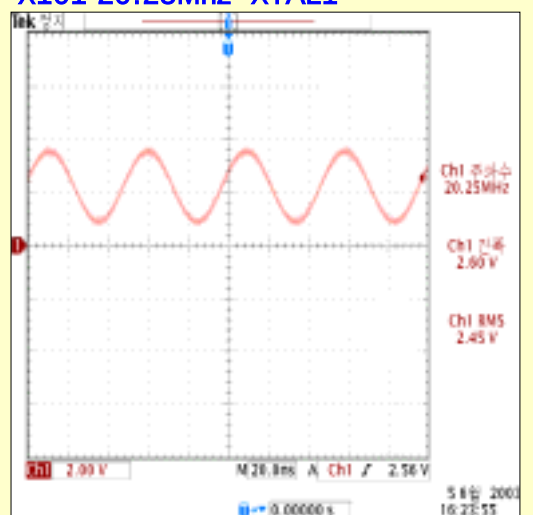
X101 20.25Mhz XTAL1
