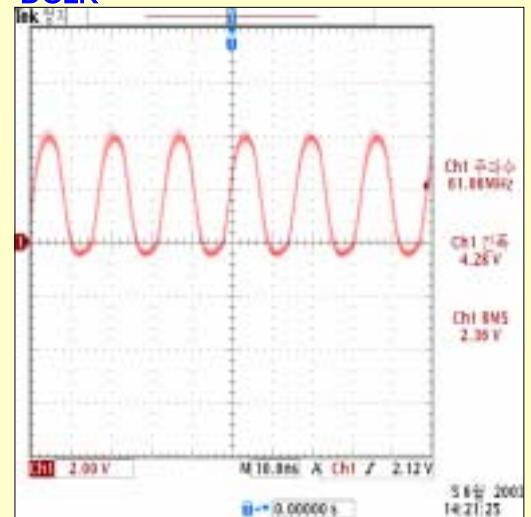
DCLK
