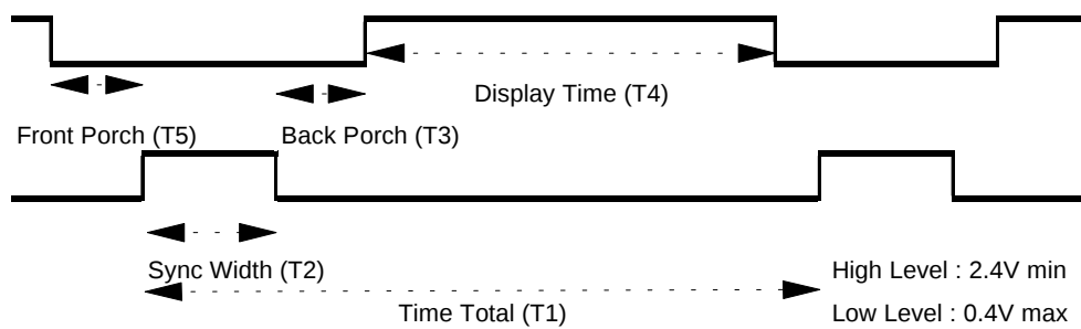
Fig. 3.02 - H-Sync
