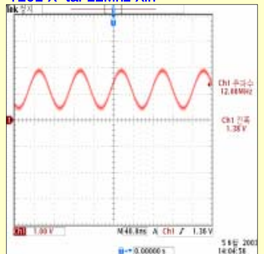
Y201 X-tal 12Mhz Xin
