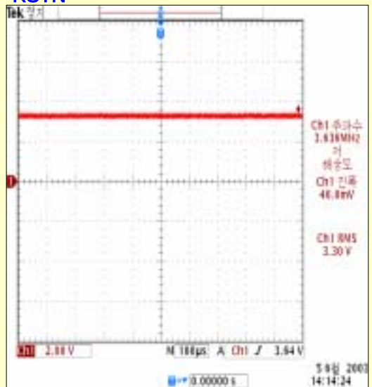
RSTN
